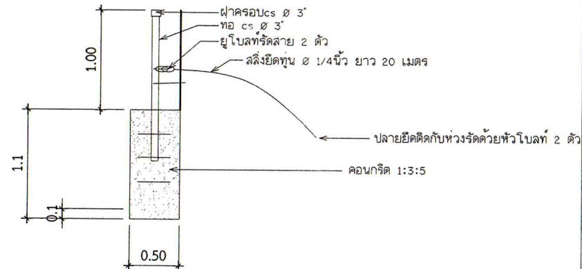
รูปขยายการติดตั้งเหล็กกันโครงท่อนล้อย
