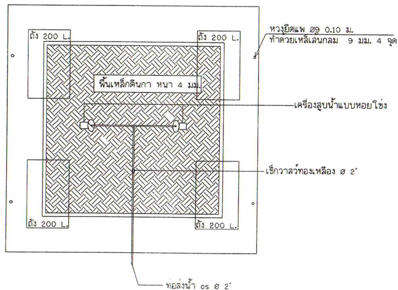
รูปแปลน ขนาด 2.00 x 2.40 เมตร
