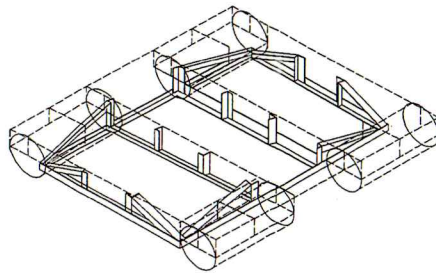
รูปขยายการติดตั้งโครงเหล็กกับท่อนล้อย
