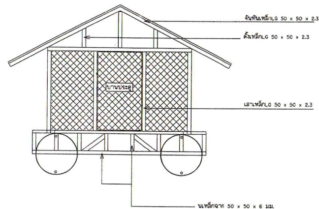
รูปด้านหน้า
