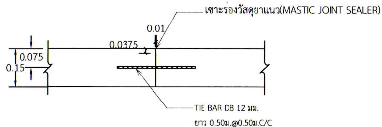
ขยายรอยต่อ LONGITUDINAL JOINT
