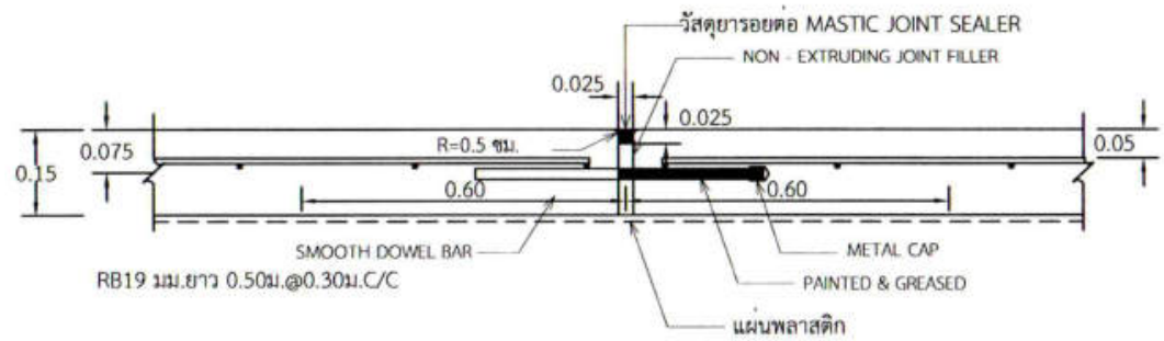
ขยายรอยต่อ EXPANSION JOINT ทุกระยะ 30.00 ม.
