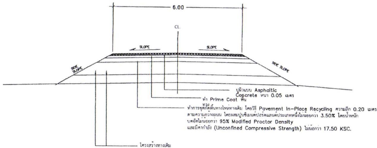
รูปตัดตามขวางโครงสร้างทาง ขนาดราสวณ NOT TO SCALE
