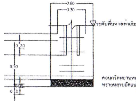
แบบขยายต่อม้อป้ายโครงการ
