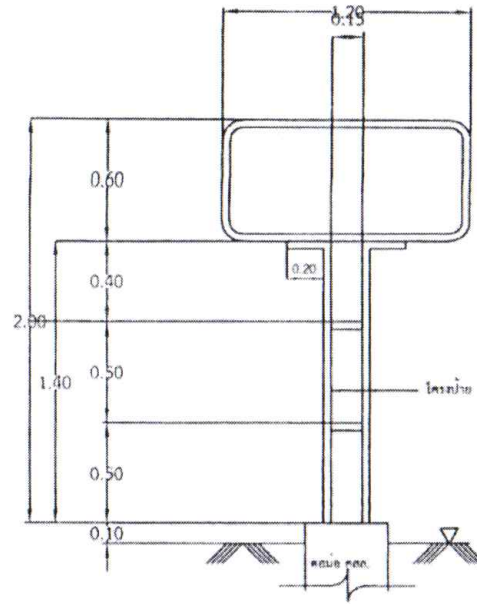
แบบป้ายโครงการ
