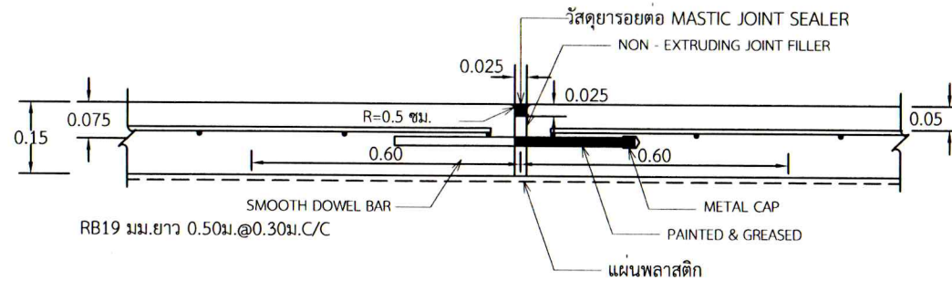
ขยายรอยต่อ EXPANSION JOINT ทุกระยะ 30.00 ม.
