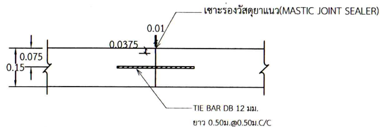
ขยายรอยต่อ LONGITUDINAL JOINT
