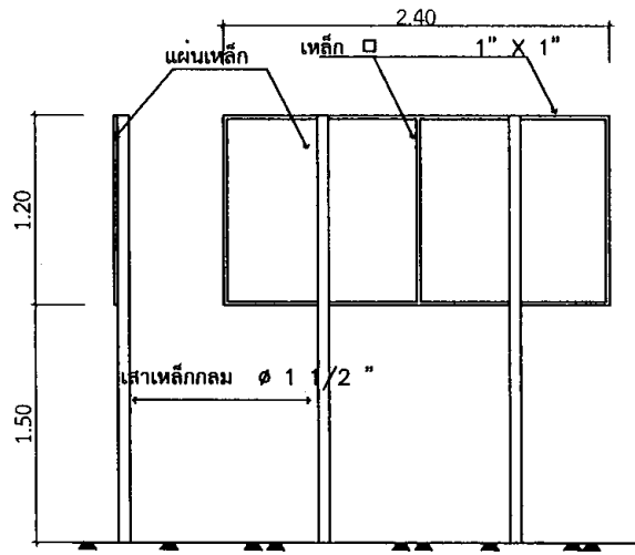
รูปด้านข้าง
