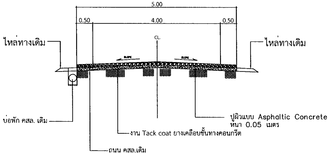
รูปตัดตามขวางโครงสร้างทาง
