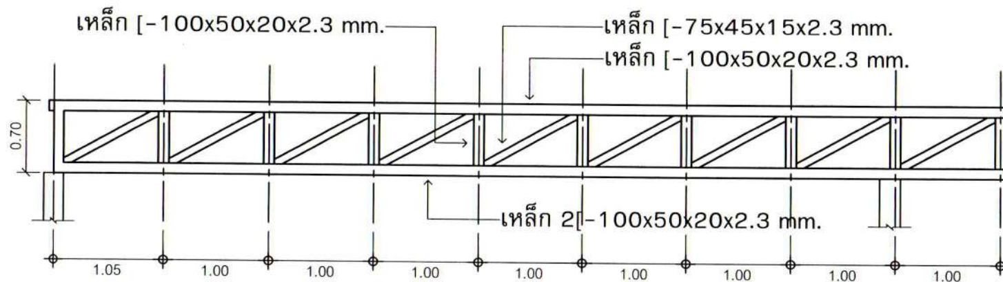
ขยาย TRUSS 1
