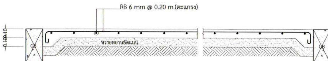
ขยายพื้น GS 1:25
