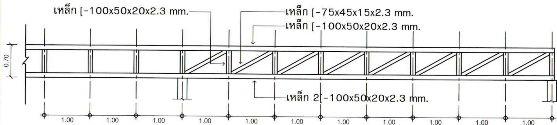
ขยาย TRUSS 2
