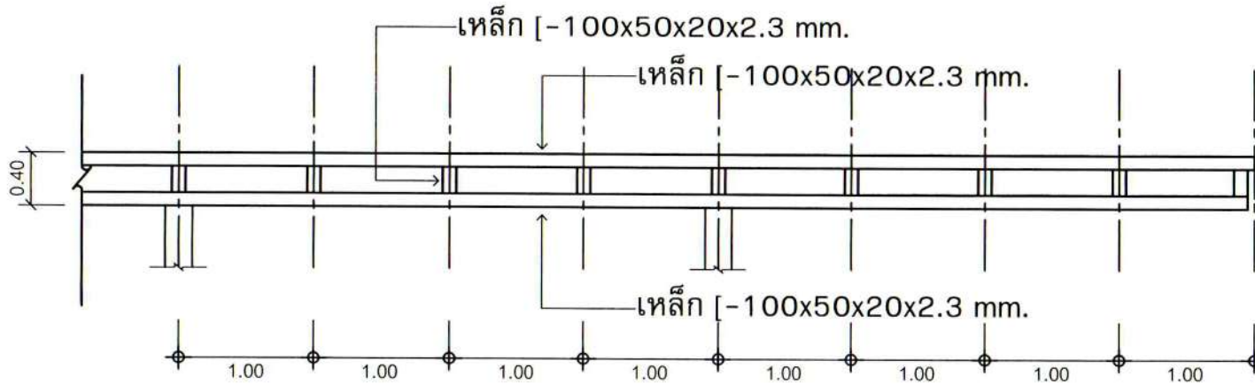
ขยาย TRUSS 3
