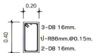
SECTION ①-①
