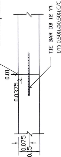
เจาะร่องวัสดุยาแนว (MASTIC JOINT SEALER)
