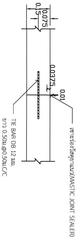
ขยายรอยต่อ LONGITUDINAL JOINT
